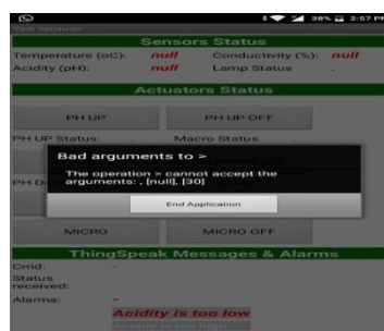
Gambar 21 Error message
