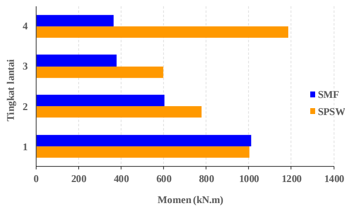
Gambar 17. Perbandingan momen pada sistem SMF dan SPSW
