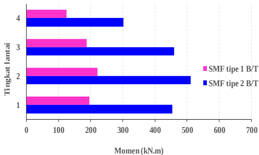
Gambar 6. Perbandingan momen di balok SMF B/T
