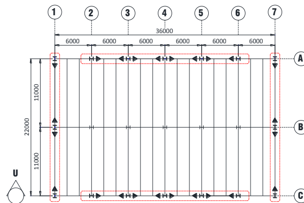
Gambar 3. Denah bangunan sistem SMF tipe 2
