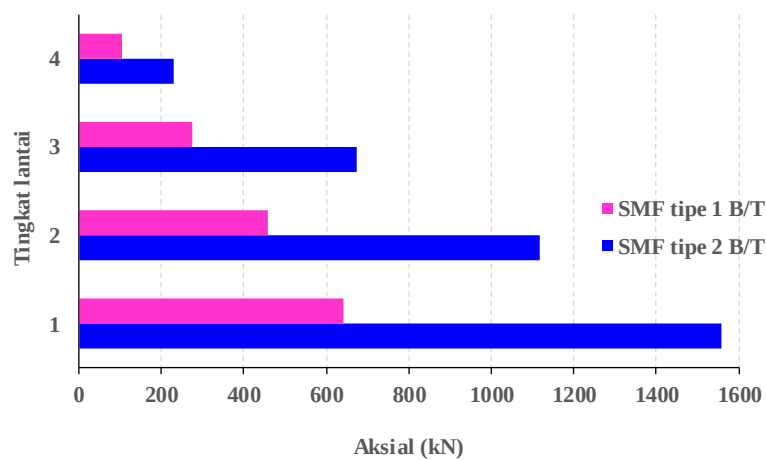
Gambar 10. Perbandingan gaya aksial di kolom SMF B/T
