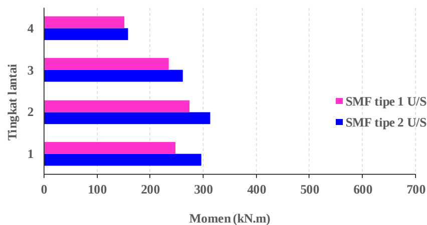
Gambar 7. Perbandingan momen di balok SMF U/S
