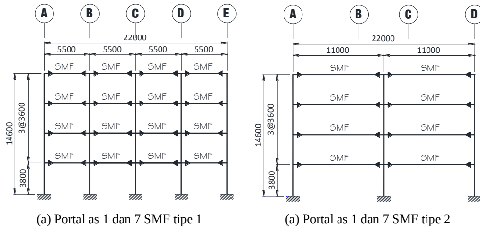
Gambar 4. Potongan melintang bangunan SMF
