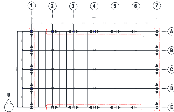
Gambar 2. Denah bangunan sistem SMF tipe 1
