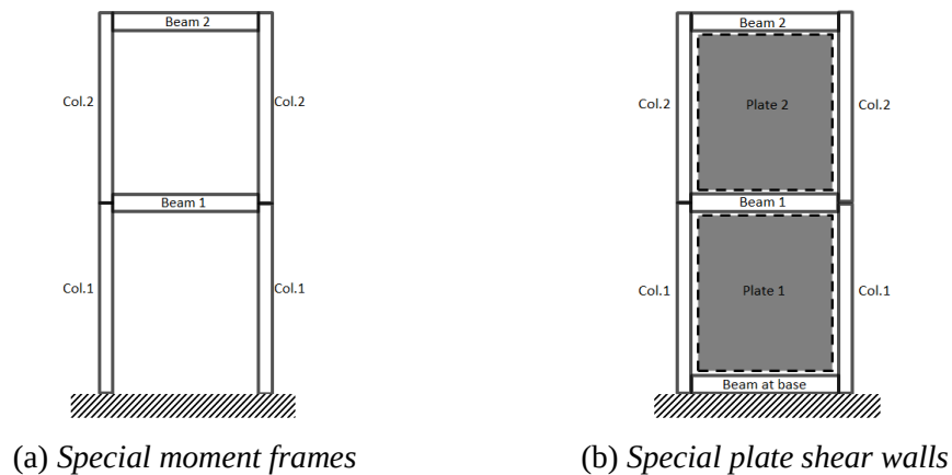
Gambar 1. Skematik sistem struktur SMF dan SPSW
