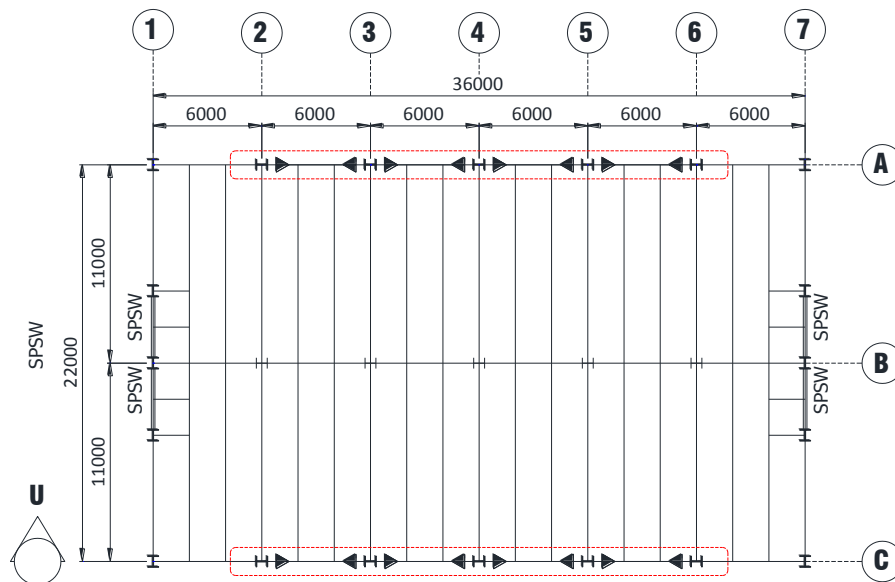
Gambar 13. Denah bangunan sistem SPSW
