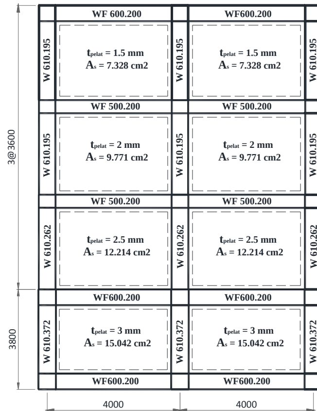
Gambar 14. Desain sistem SPSW
