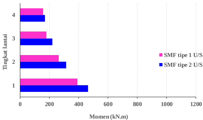
Gambar 9. Perbandingan momen di kolom SMF U/S
