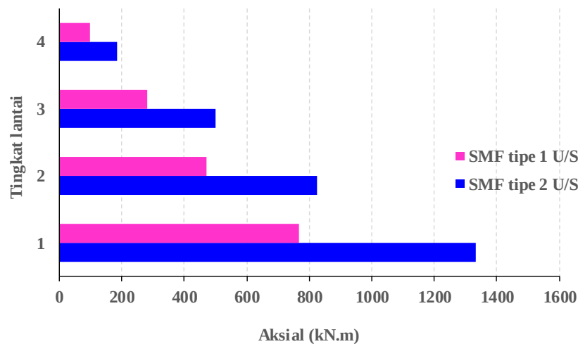
Gambar 11. Perbandingan gaya aksial di kolom SMF U/S
