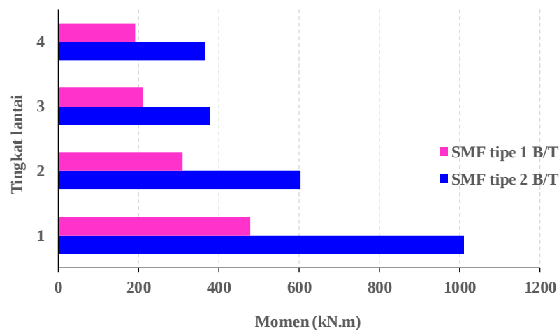
Gambar 8. Perbandingan momen di kolom SMF B/T
