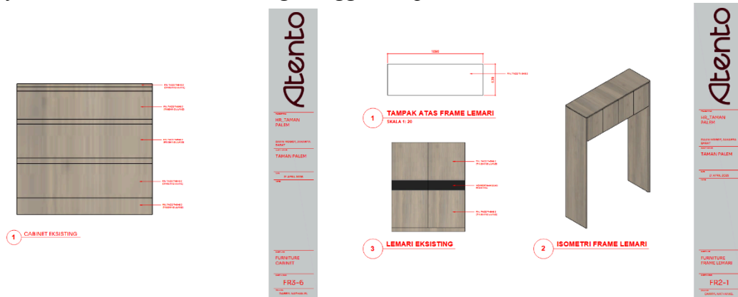
Gambar kerja lemari dan cabinet eksisting mengganti lapisan HPL
