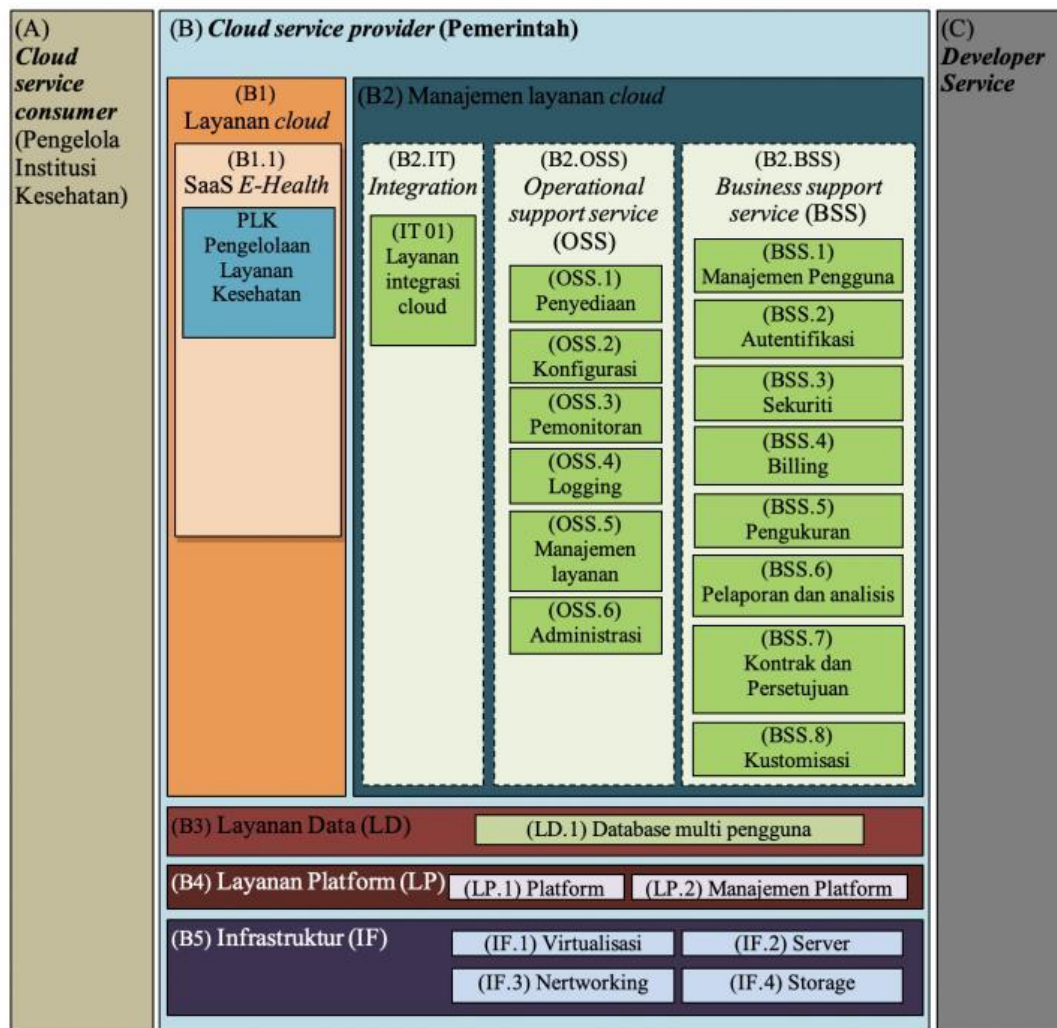
Gambar 3 Arsitektur SaaS
