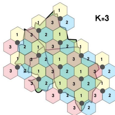
Gambar 2 Pemetaan Site dengan Frequency Reuse k=3
